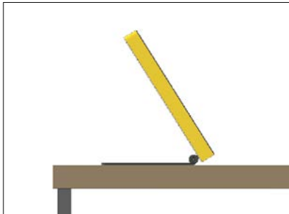
STANDMODELL KLASSISCH
