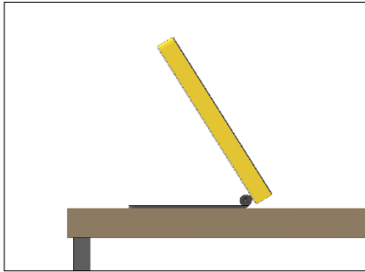
STANDMODELL KLASSISCH
